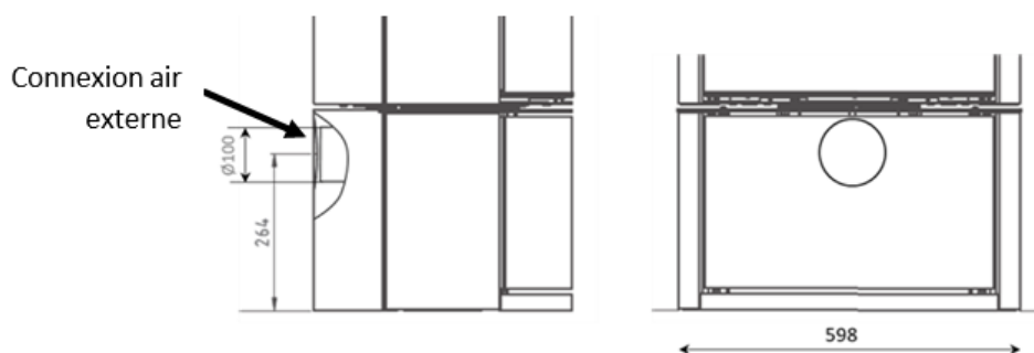
Figure 4 – Connexion à l'air extérieur
