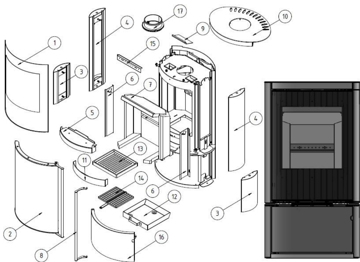
Figure 2 – Composants du poêle
