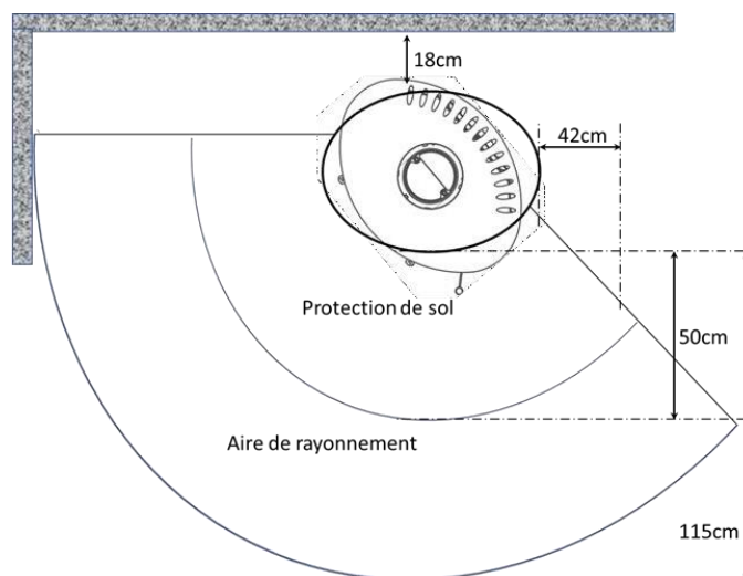
Figure 3 – Distances de sécurité
