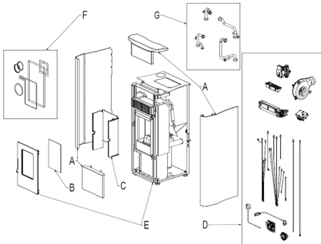
Fig. 1 - Dessin éclaté
