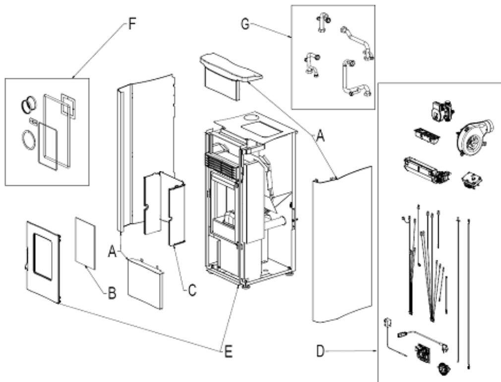
Fig. 1 - Dessin éclaté
