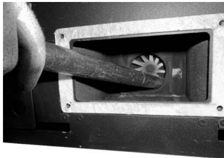
Fig. 95 - Aspirer les cendres
