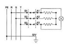
SCHEMA ÉLECTRIQUE (TRIPHASE)
